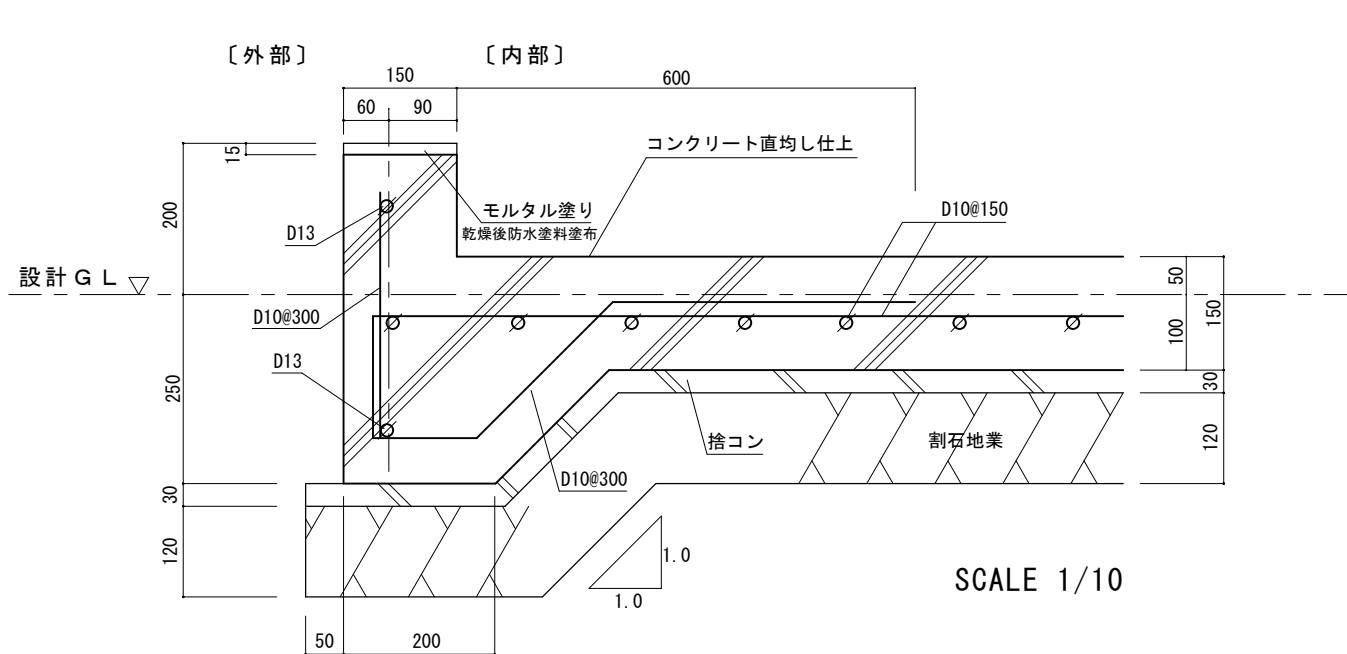
スライディングルーフ用 布基礎
