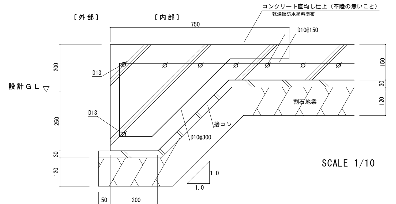
スライディングルーフ用 べた基礎
